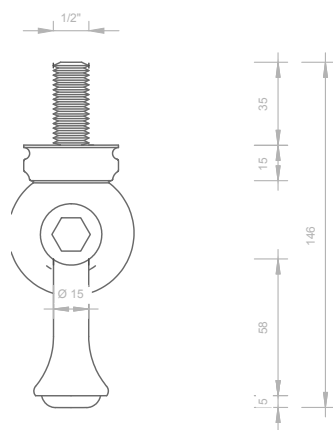
01 PLAN - GLOBE TAPS - HOT 1 : 2
