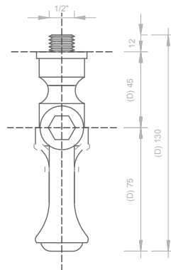
01 PLAN - BIB TAPS 1 : 2
