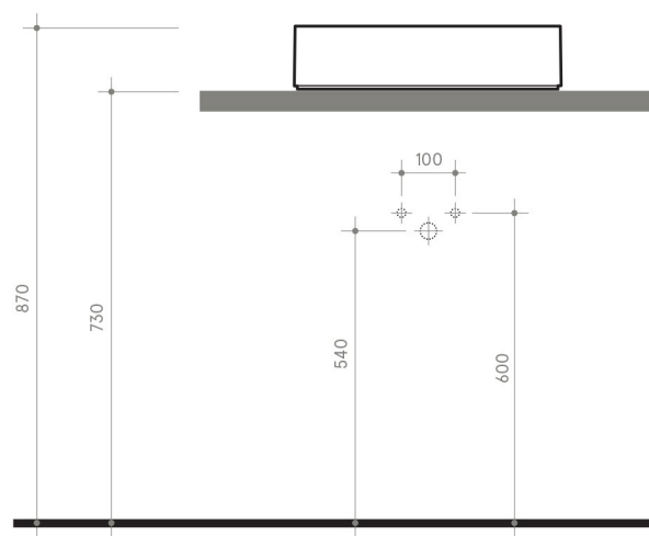
Appoggio / sit-on
