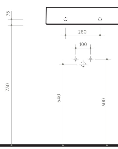
Sospeso / wall-hung
